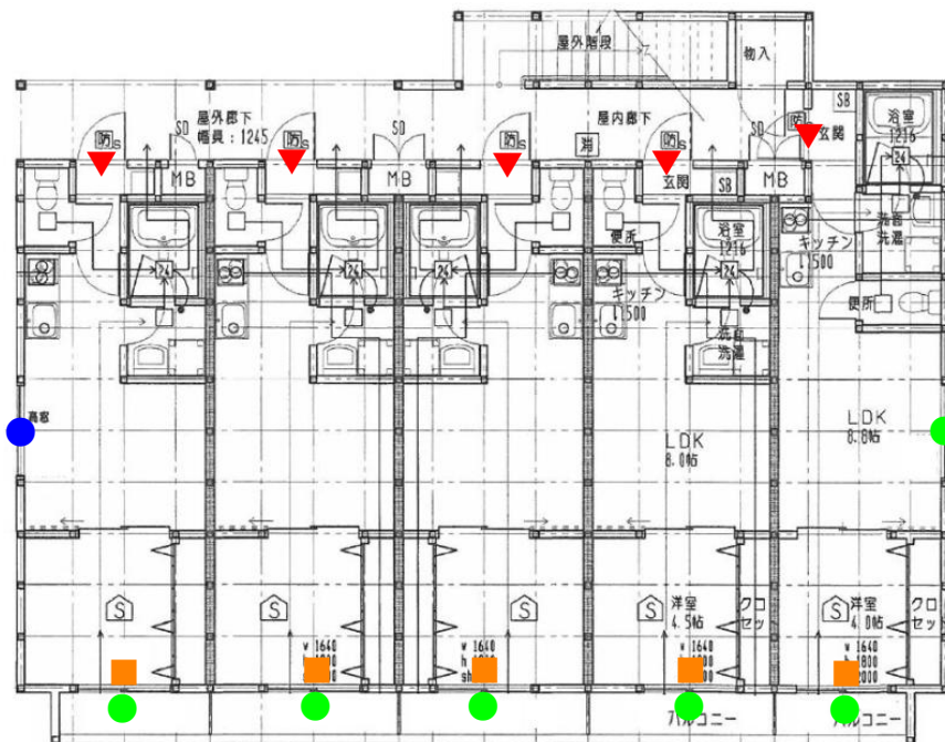
1階平面図
